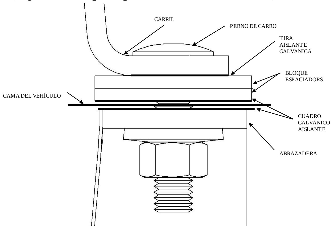
Figura 5 – Bloque Espaciador Encima de la Cama
